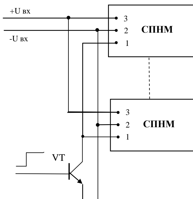
Рисунок Н.2 – Управление одновременно несколькими модулями питания
