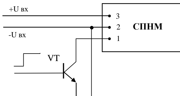
Рисунок Н.1 – Управление одиночным модулем питания
