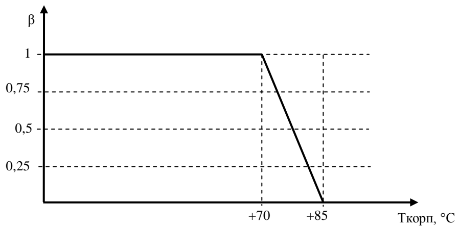
Рисунок Л.1 – Зависимость коэффициента нагрузки ( \beta ) модуля питания от температуры корпуса модуля питания.
